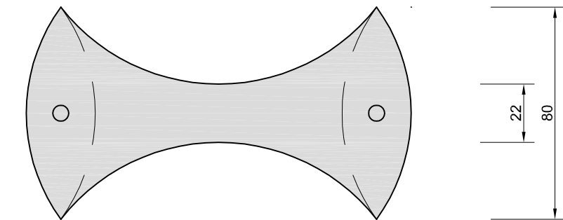
Griff Ansicht Oben 1:2
